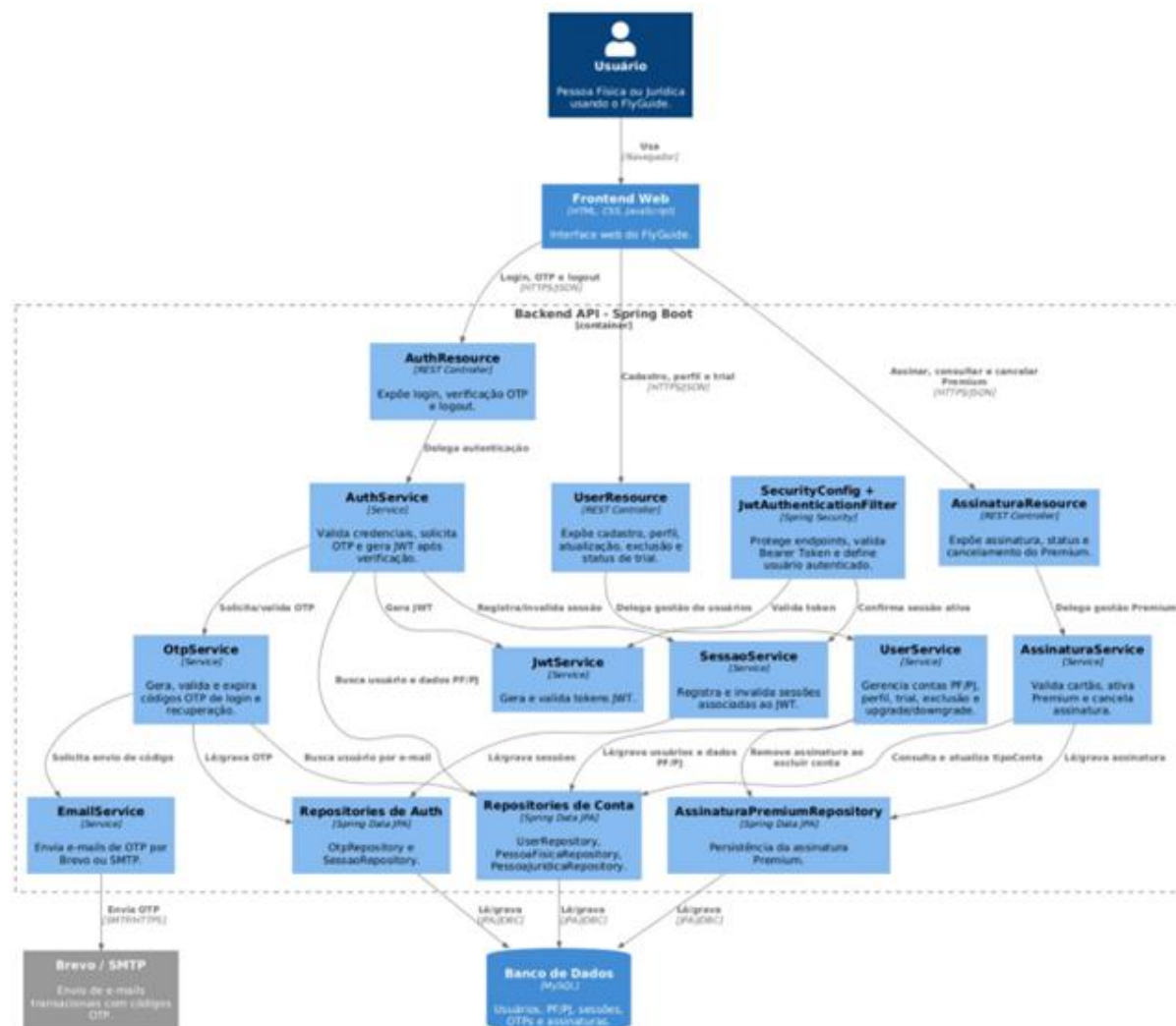
Figura 29 - Modelo C3 sobre fluxos de Usuários, Autenticação e Premium
