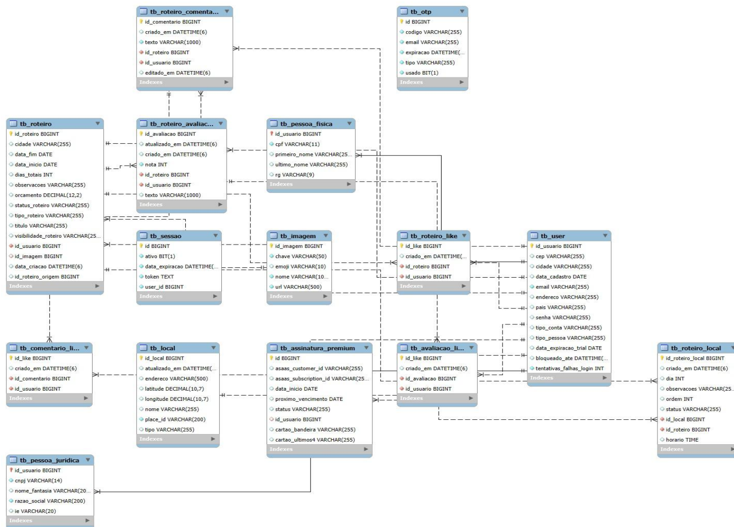
Figura 26 - Modelo físico DER
