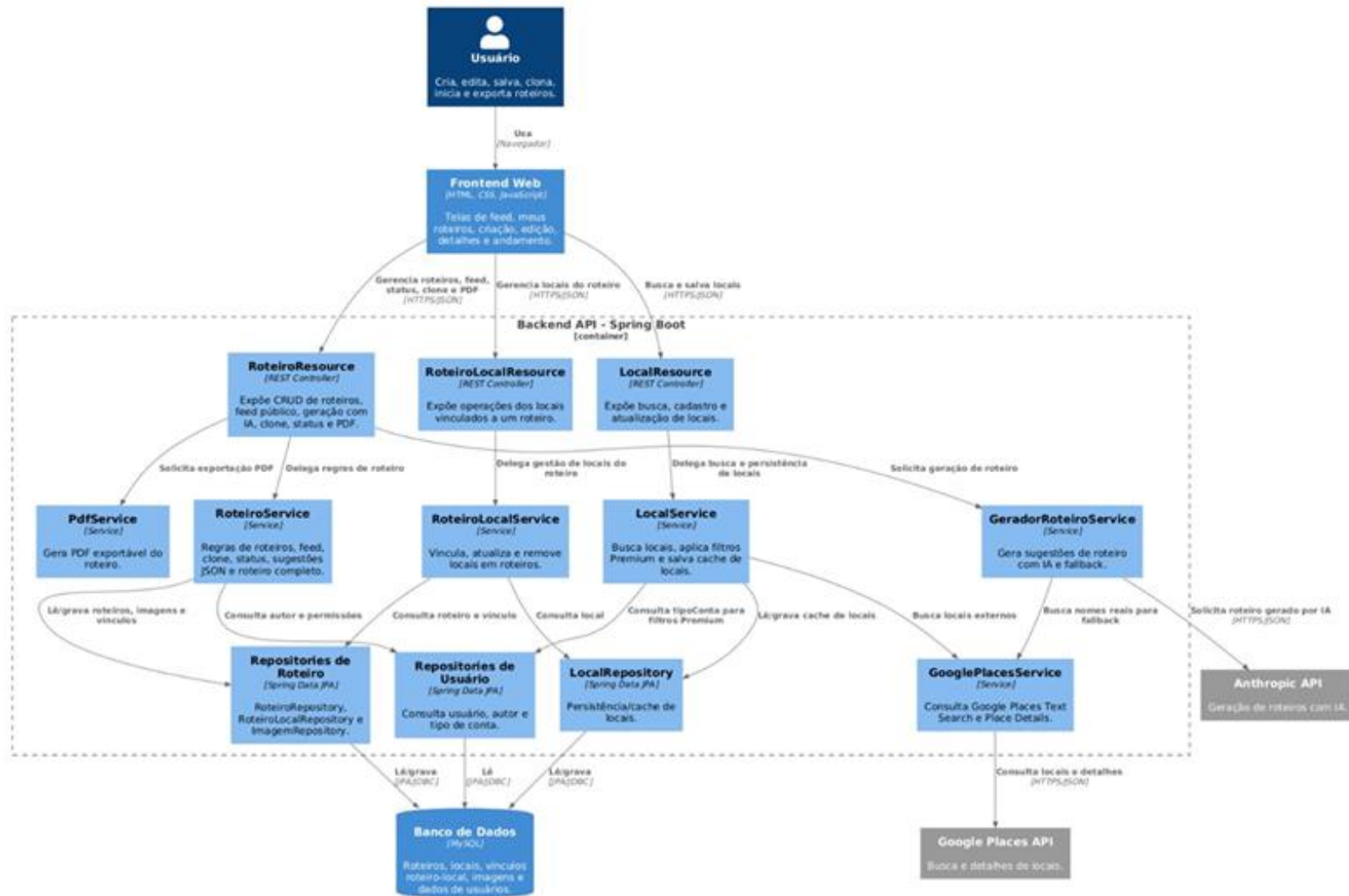
Figura 30 - Modelo C3 sobre componente de Roteiros e Locais
