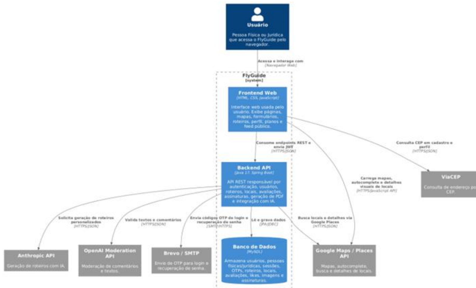
Figura 28 - Modelo C2 sobre o sistema
