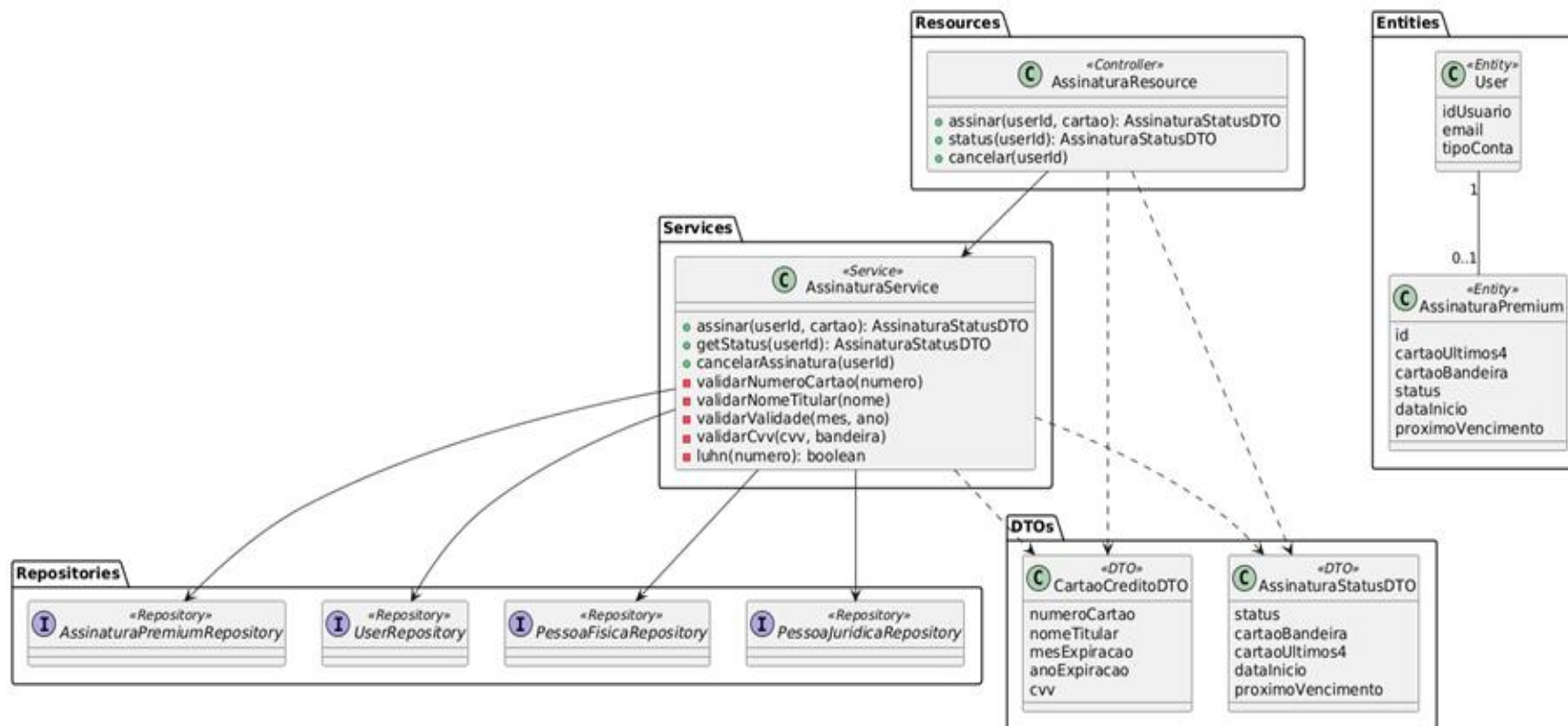
Figura 38 - Modelo C4 sobre componentes de Assinatura Premium
