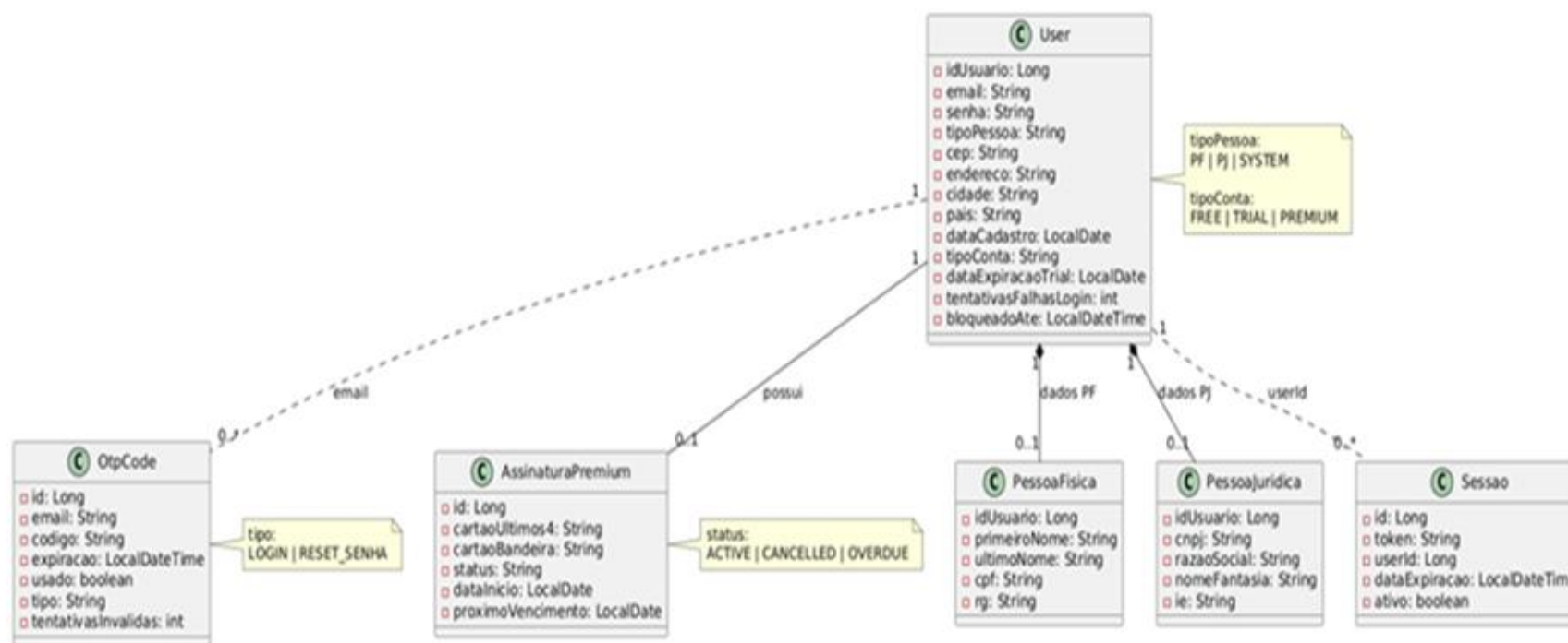
Figura 6 - Diagrama de Classes – Serviços de Usuários, Autenticação e Premium
